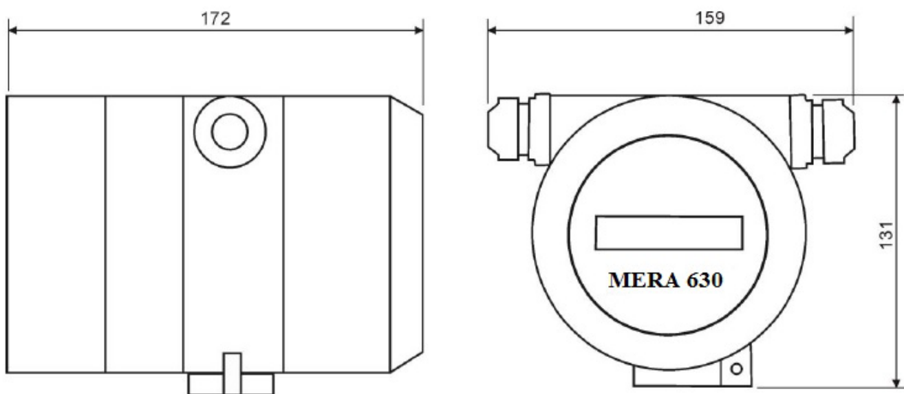
Рис. 3е Внешние размеры преобразователя MERA 630
