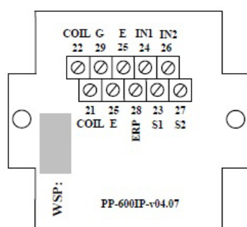
Соединительная панель датчика тип PP-600IP-v04.07
