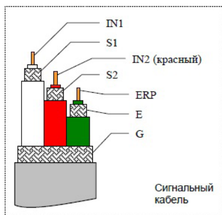
Рис. 3ж внешнее соединение датчика и преобразователя
