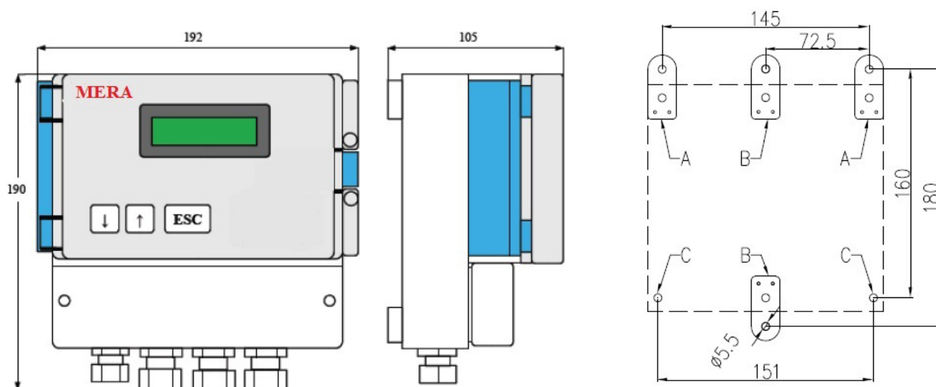
Рис. 3в Внешние размеры преобразователя MERA 600
