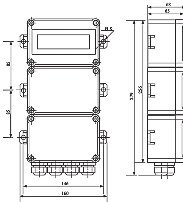
Рис.3а Габаритные размеры преобразователя MERA 600Ex (корпус 0В 3-Р154-0000333)
