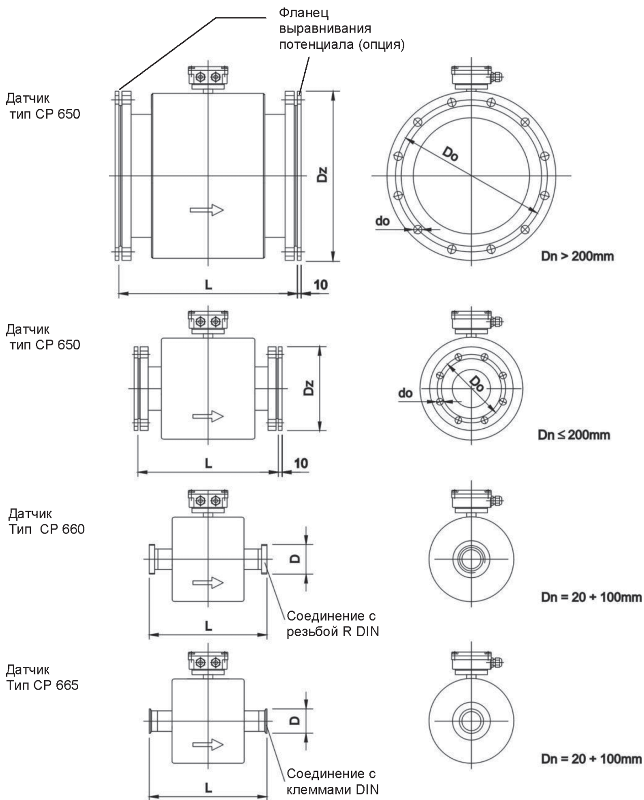
Рис.1 Размеры датчиков
