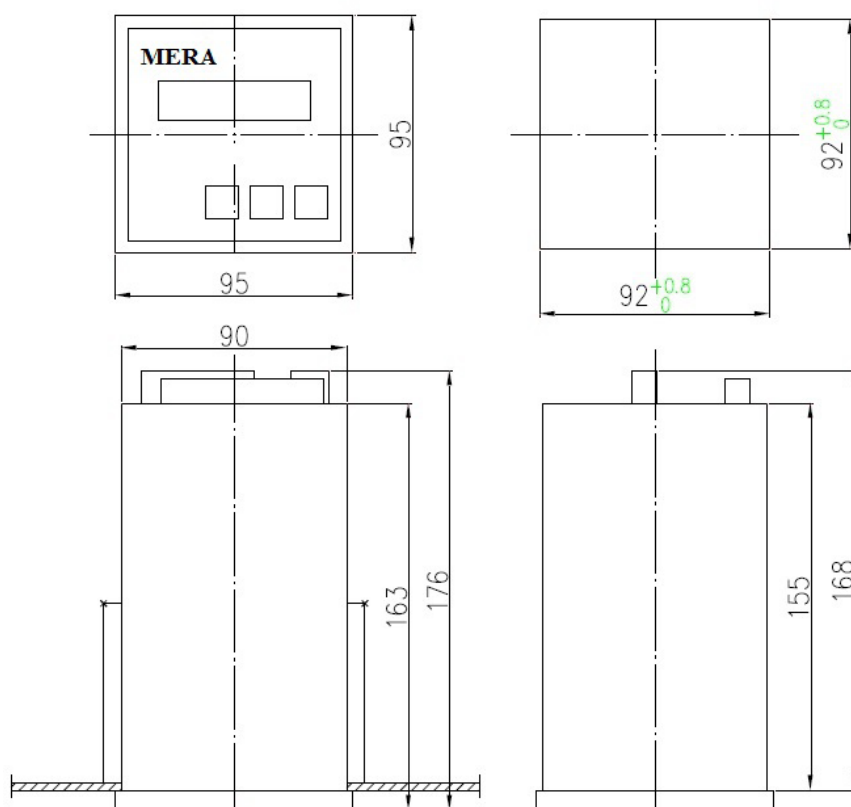
Рис. 3д Внешние размеры преобразователя MERA 620
