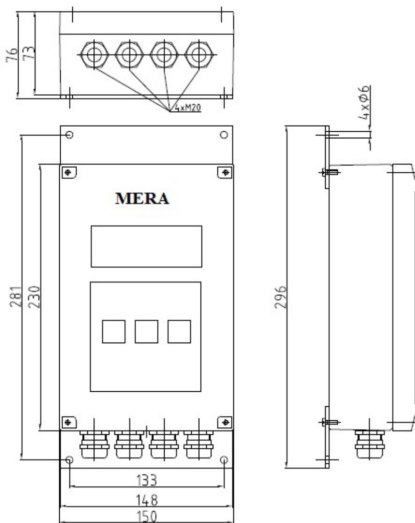
Рис. 3г Внешние размеры преобразователя MERA 610
