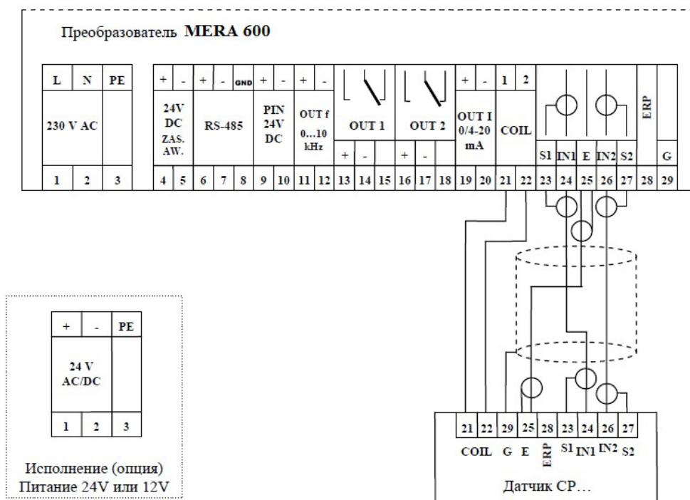
Рис. 3ж внешнее соединение датчика и преобразователя
